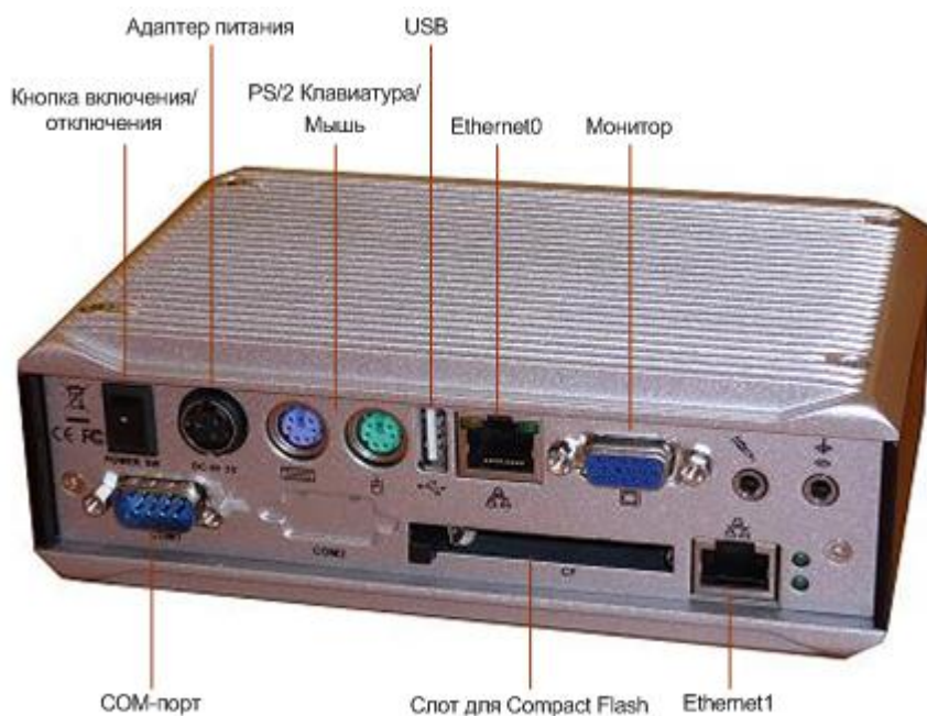
Рисунок 2: Задняя панель ПАК HW100 G1
