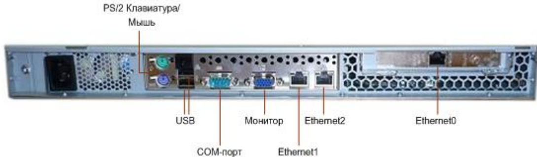
Рисунок 5: Задняя панель ПАК HW1000 G1
