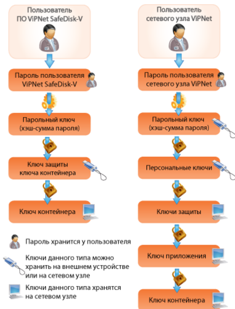
Рисунок 71: Схема иерархии защиты ключа контейнера в ПО VIPNet SafeDisk-V, интегрированного с VIPNet Client
