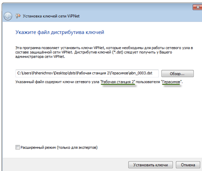
Рисунок 11: Выбор файла дистрибутива ключей
