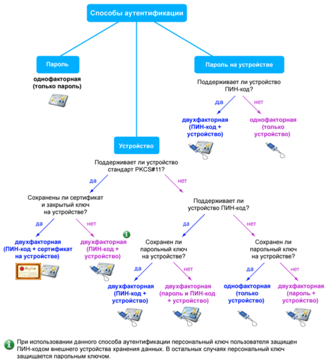
Рисунок 17: Схема соответствия между факторами и способами аутентификации
