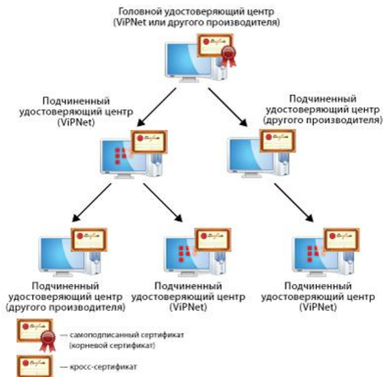
Рисунок 141: Иерархическая модель доверительных отношений
