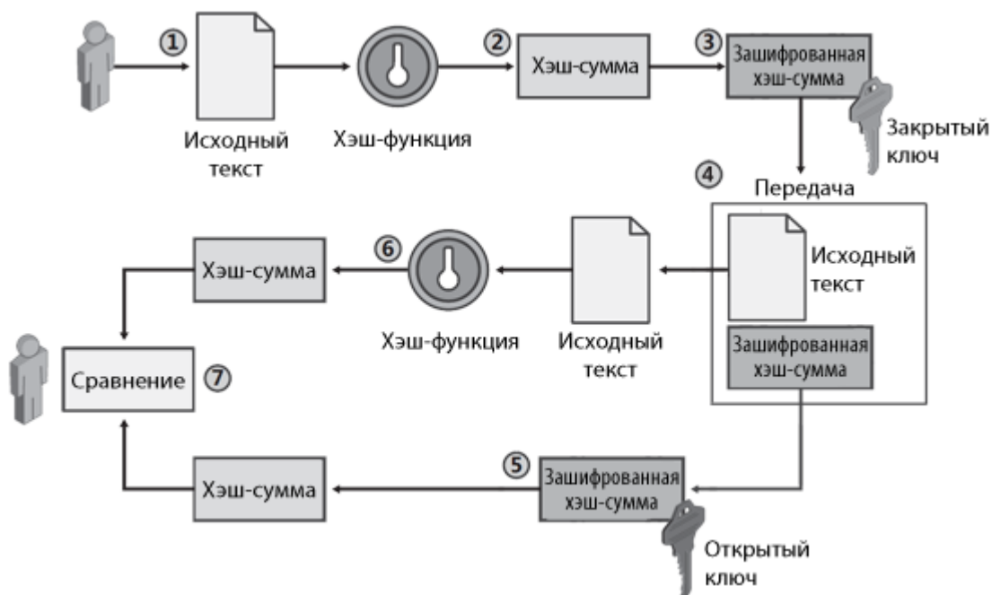
Рисунок 137: Применение хэш-функции и асимметричного алгоритма в электронной цифровой подписи
