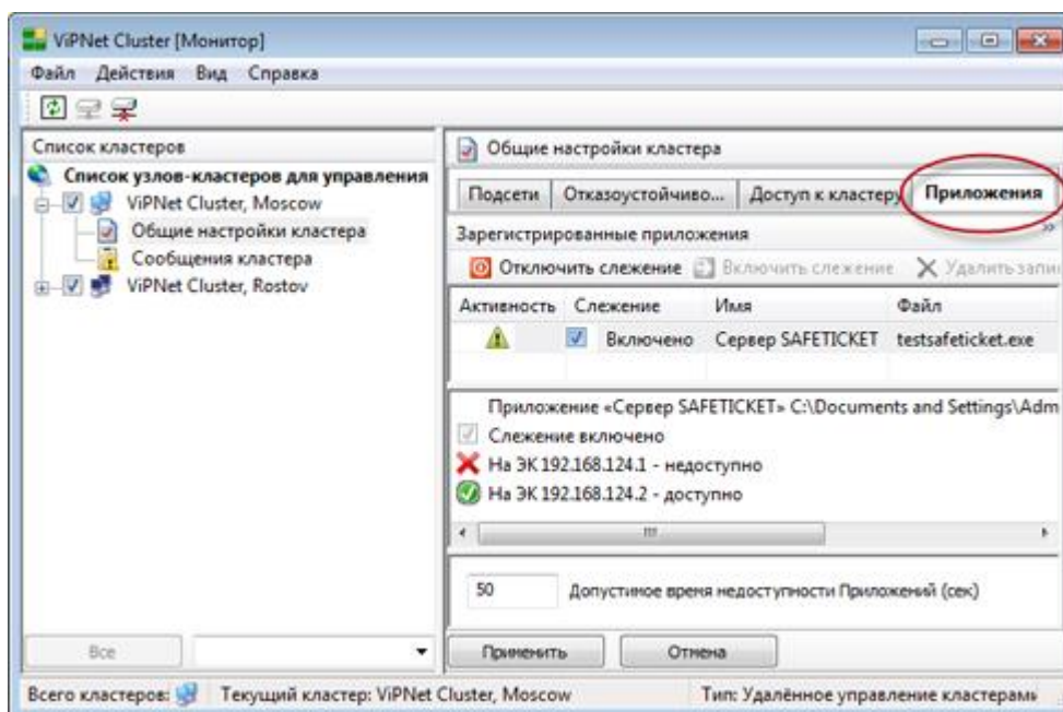
Рисунок 183: Настройка параметров контроля приложений в ViPNet Cluster Монитор
