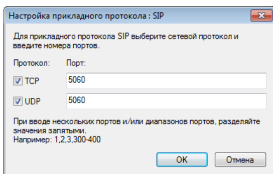
Рисунок 70: Настройка параметров обработки прикладного протокола
