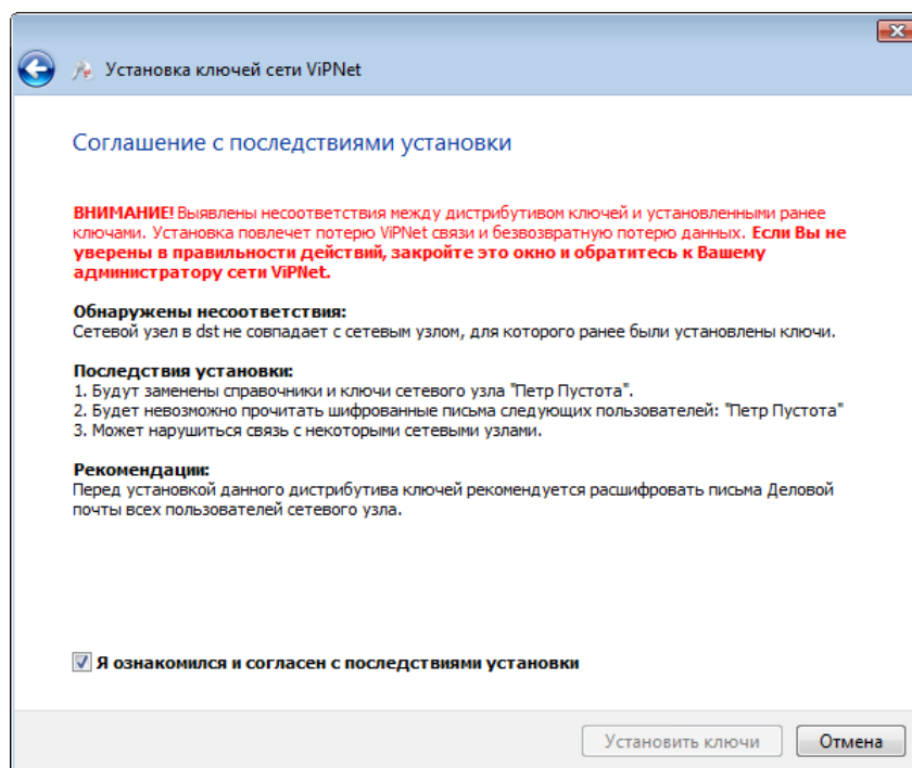
Рисунок 14: Обнаружено несоответствие между дистрибутивом и текущими ключами на узле
