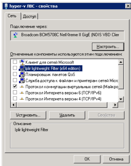
Рисунок 164: Настройки физического интерфейса, подключенного к виртуальной сети Hyper-V
