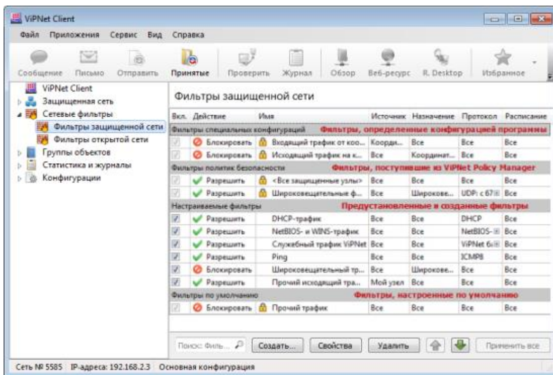
Рисунок 171: Отображение сетевых фильтров в программе ViPNet Монитор
