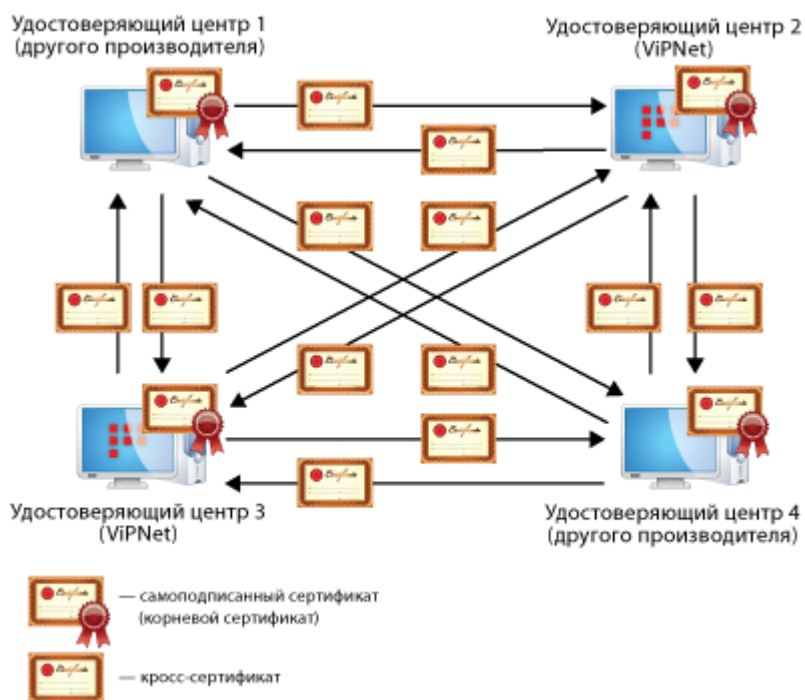
Рисунок 142: Распределенная модель доверительных отношений
