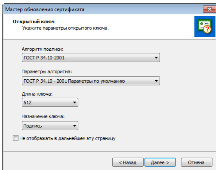
Рисунок 112: Выбор алгоритма и его параметров
