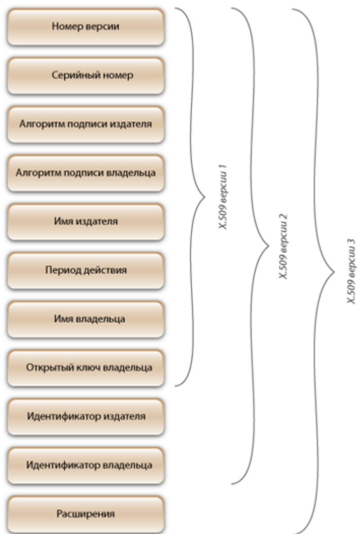
Рисунок 139: Структура сертификата, соответствующего стандарту X.509 версий 1, 2 и 3
