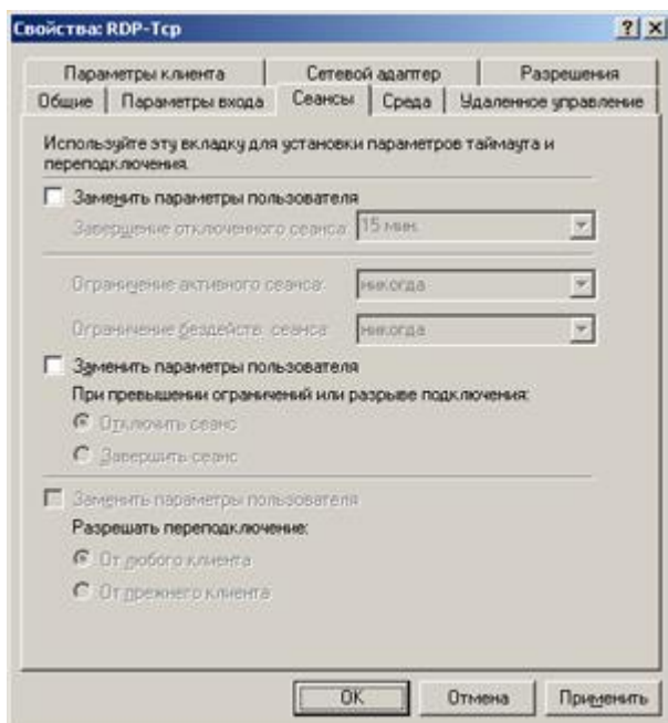
Рисунок 92: Верные настройки терминального сервера
