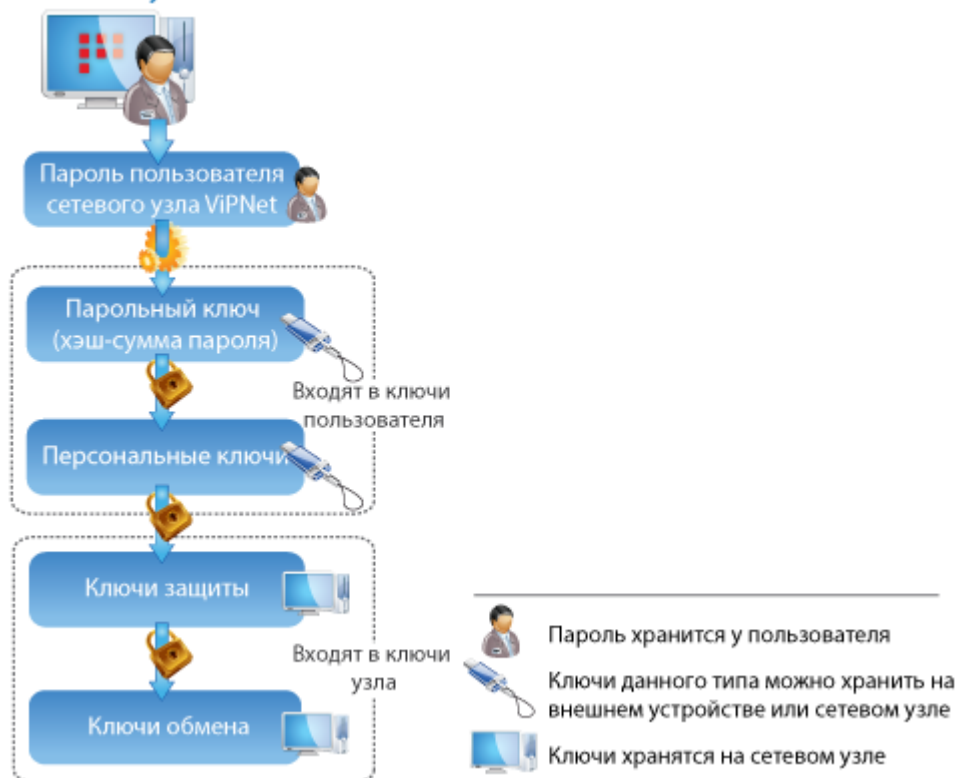
Рисунок 150: Иерархия защиты ключей обмена на сетевом узле
